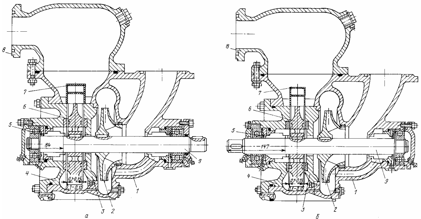
Рис. 1. Конструкция электронасоса 1CЦЛ-20-24Г:
