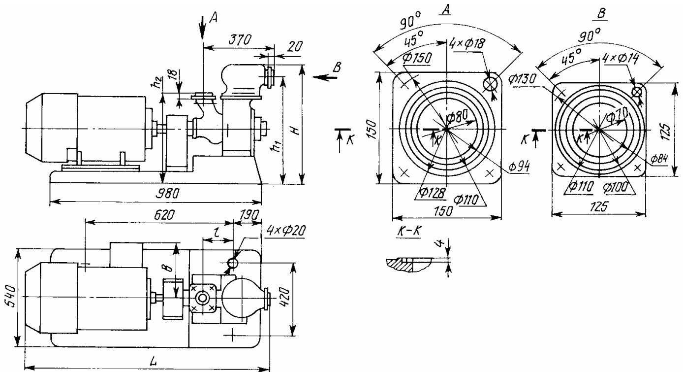
Рис. 4. Общий вид, габаритные, присоединительные размеры и масса электронасосного агрегата 1АСЦЛ-20-24Г на железобетонной фундаментной плите
